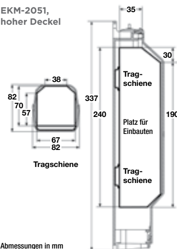
Positionsmöglichkeiten der Tragschiene
