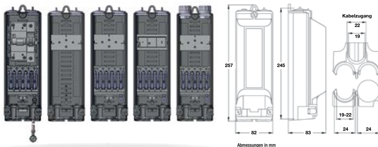
EKM-2050-5S-FILS/LS-DE01 EKM-2050-1R/A EKM-2050F-5S-1R/A EKM-2050-5S-1R/D EKM-2050FH-5S-1R/A
