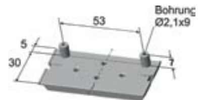
Typ B, mit Domen
