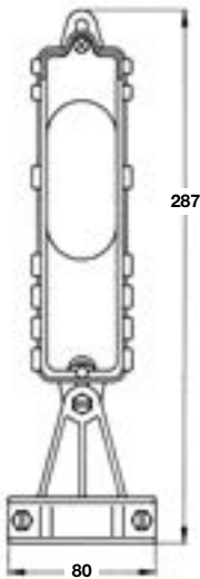
E 214 mit Zugentlastung
