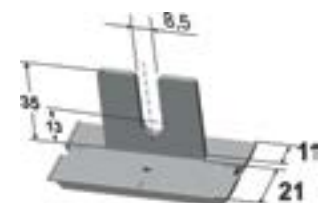
Typ C, mit Flansch
