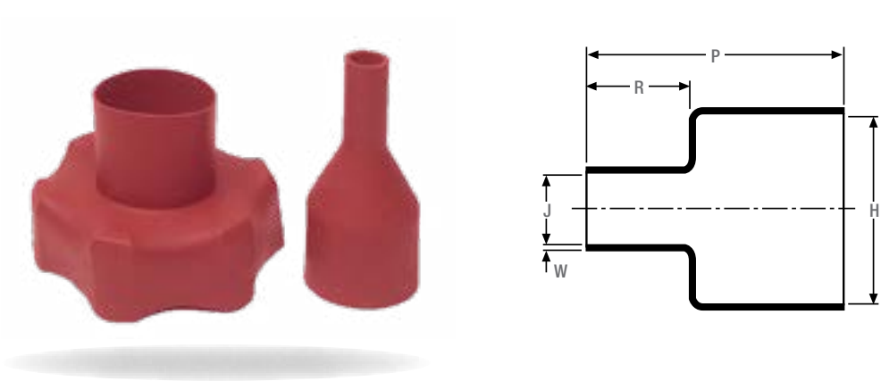
208R066 – Formteil zur Abdeckung an einem Ventilableiter, Haube nach unten offen
