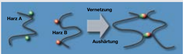
Bild 1 Schematische Darstellung der Reaktion bei GUROFLEX-N
